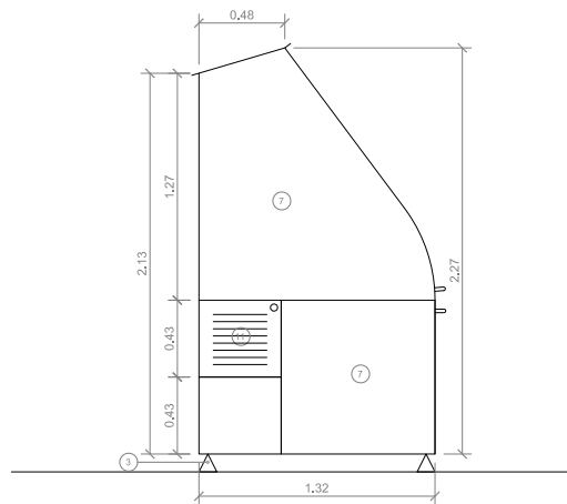
ALZADO LATERAL IZQUIERDO
