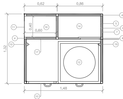
PLANTA GENERAL CERRADO
