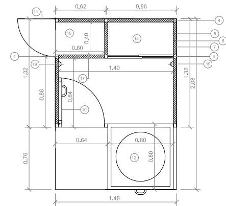
PLANTA GENERAL ABIERTO
