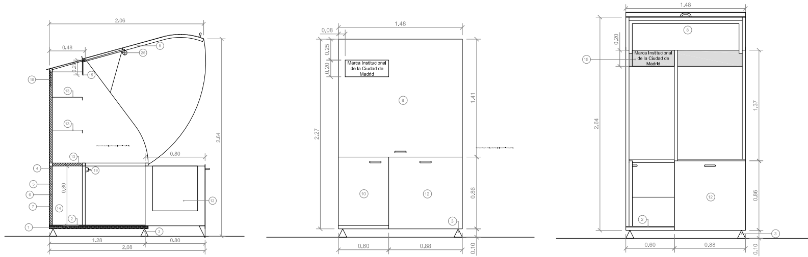
SECCIÓN DERECHA ABIERTO
