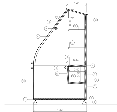
ALZADO LATERAL DERECHO
