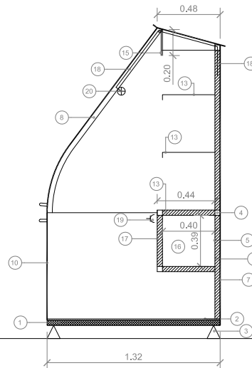
SECCIÓN IZQUIERDA CERRADO
